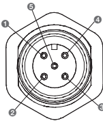
<Moduł LED>
