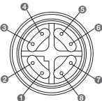
[Schemat styków złącza czytnika kodów kreskowych]
