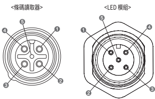
[條碼讀取器連接器的腳位圖]
