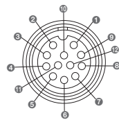
[條碼讀取器連接器的腳位圖]
