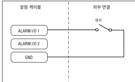
<ALARM I/O 1을 입력단자로 설정시>
