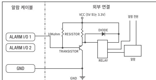
<ALARM I/O 1을 출력단자로 설정시>
