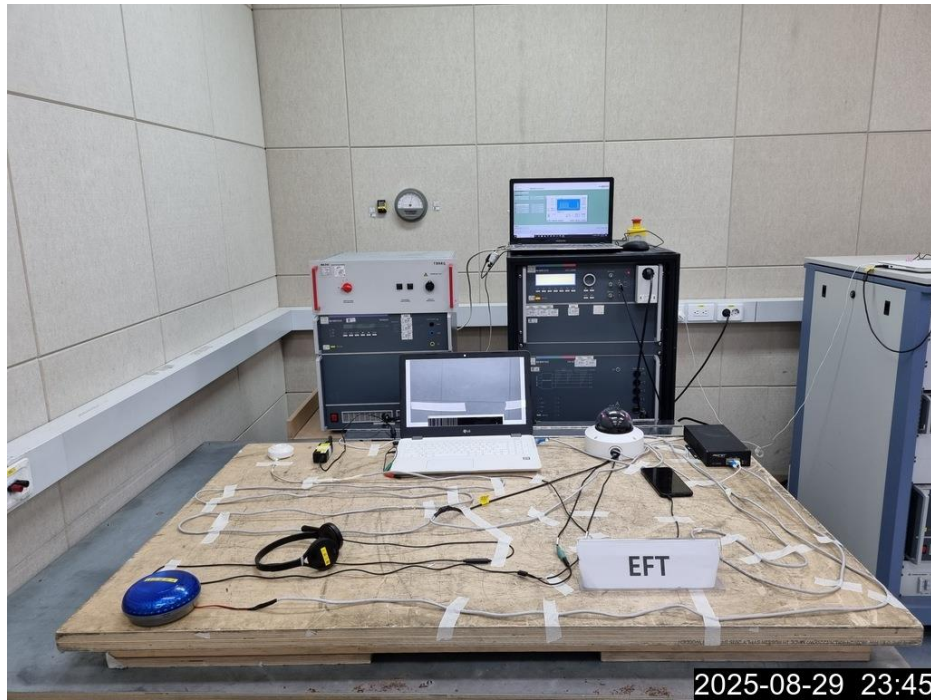
<전기적 빠른 과도 현상>
