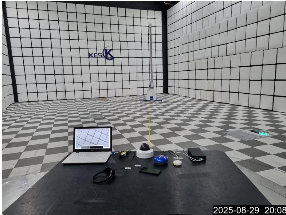
<방사성 방해-전면>
