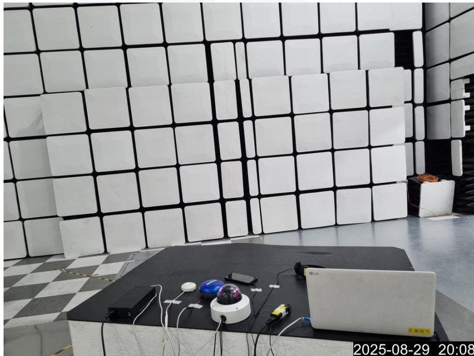
<방사성 방해-후면>
