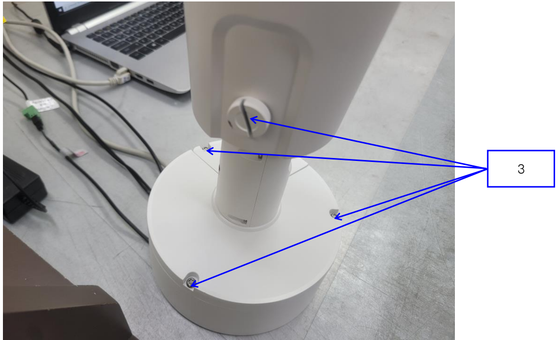
[시험기자재]_DC 모드
