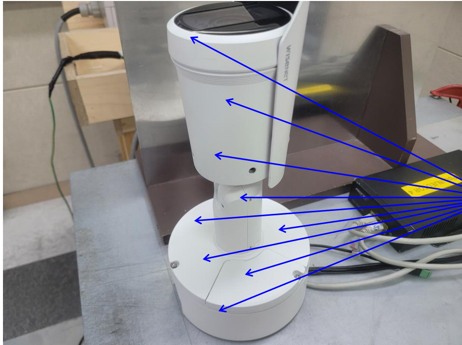
[시험기자재]_PoE 모드
