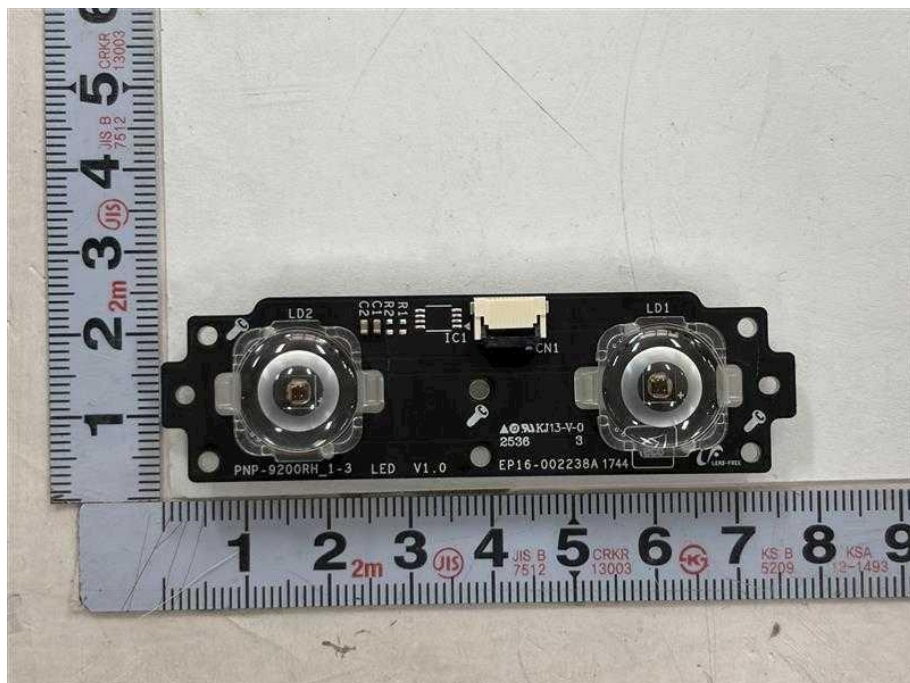
<Photo 4> IR LED 보드
