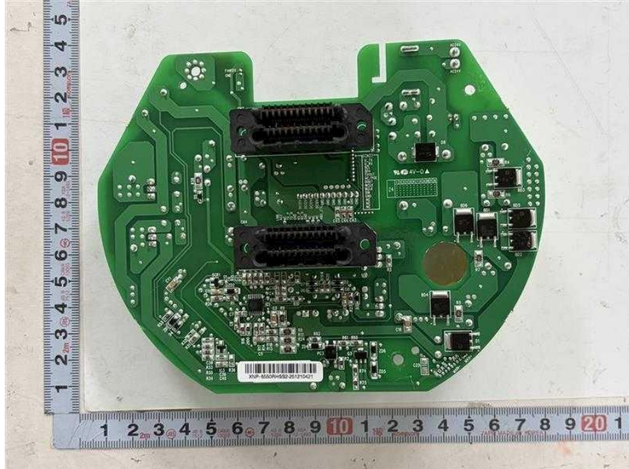
<Photo 14> PoE 보드
