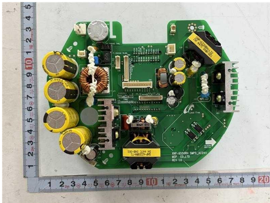
<Photo 12> Power 보드
