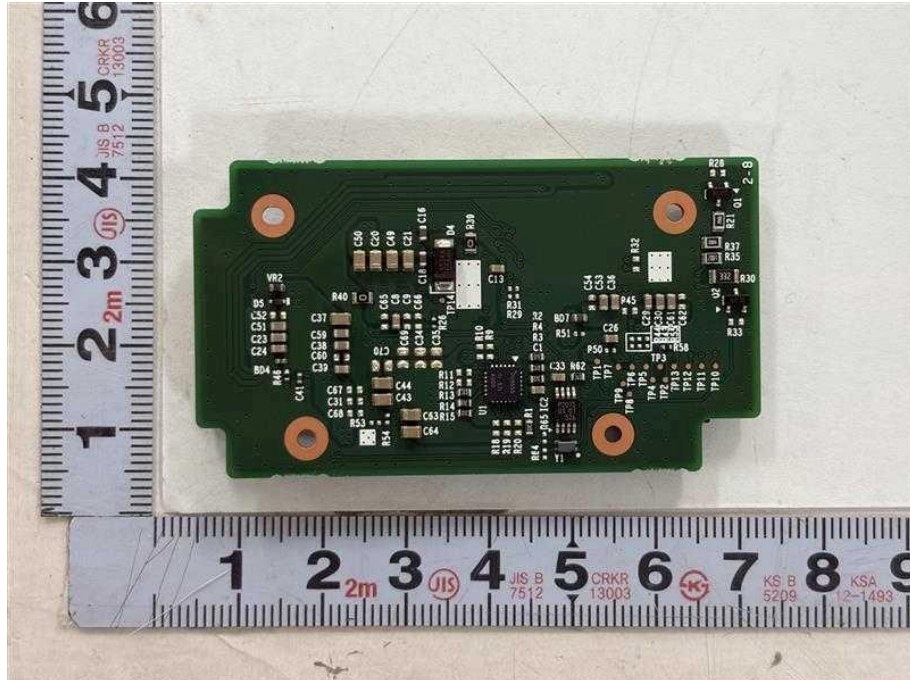
<Photo 8> Network 보드
