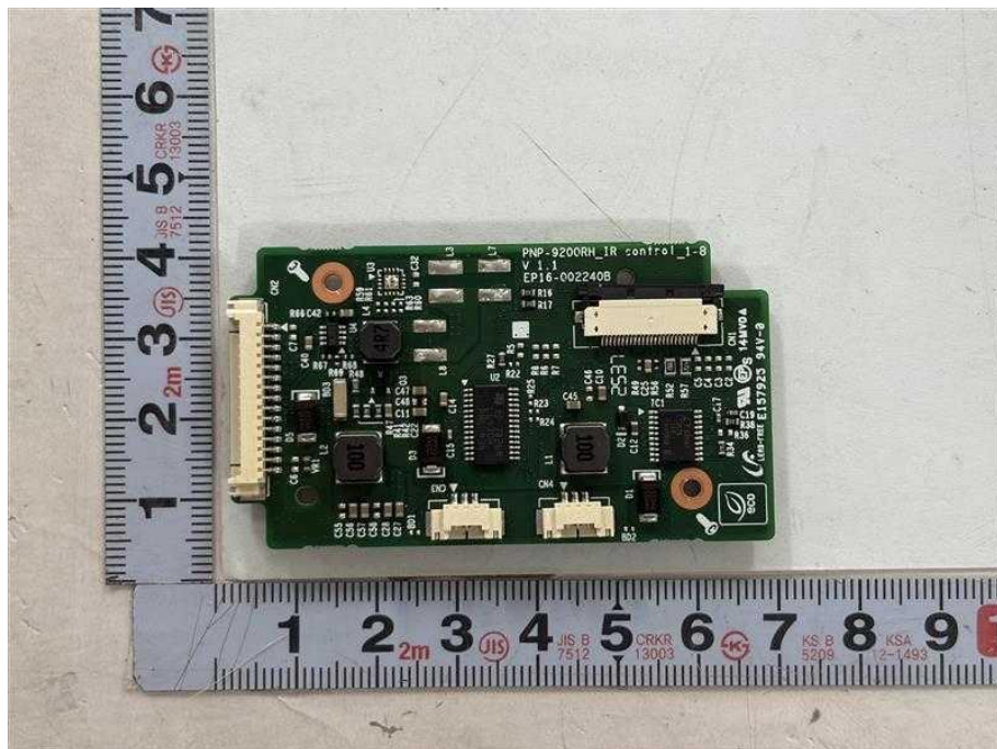
<Photo 6> IR Control 보드
