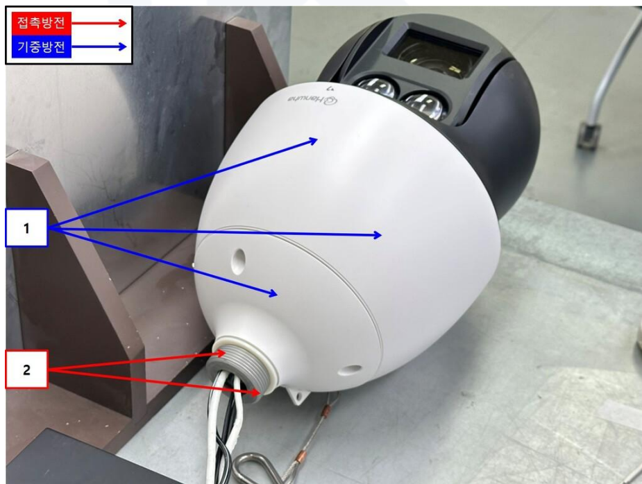
<정전기 인가부위-2> Mode 1
