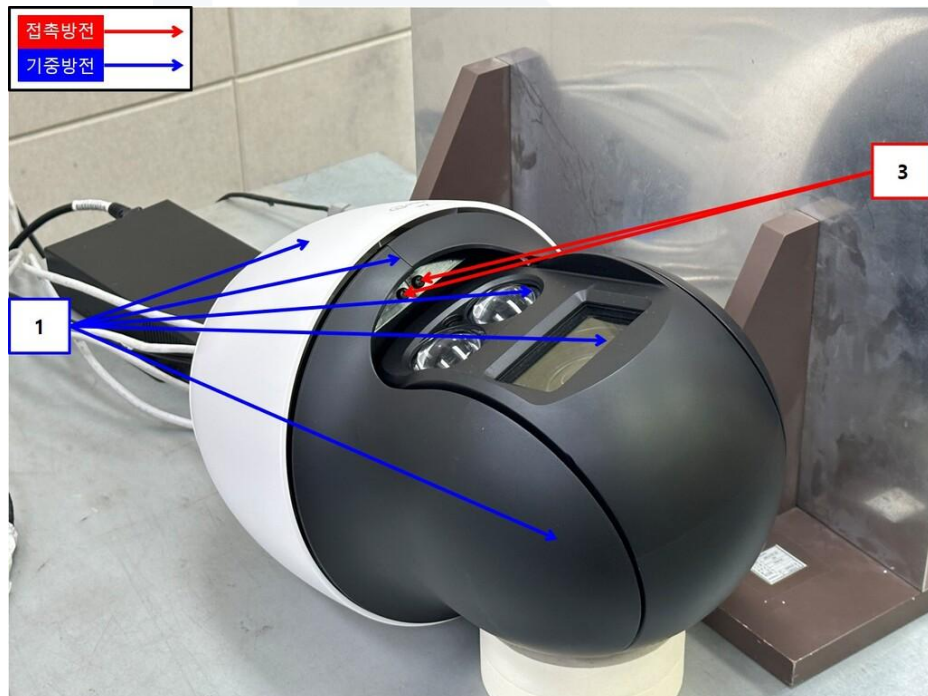
<정전기 인가부위-1> Mode 2
