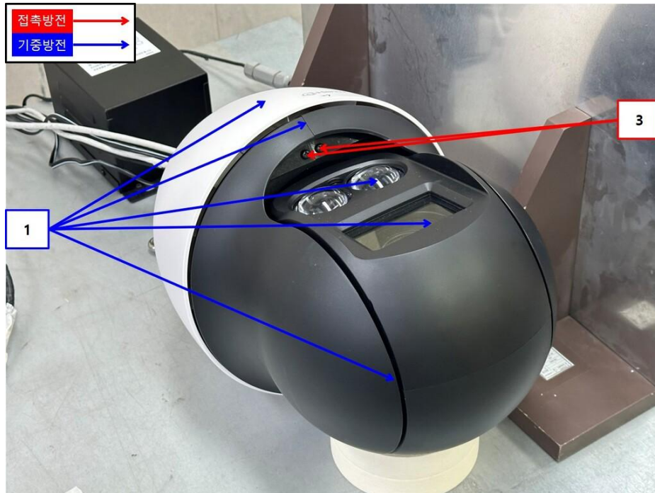
<정전기 인가부위-1> Mode 1
