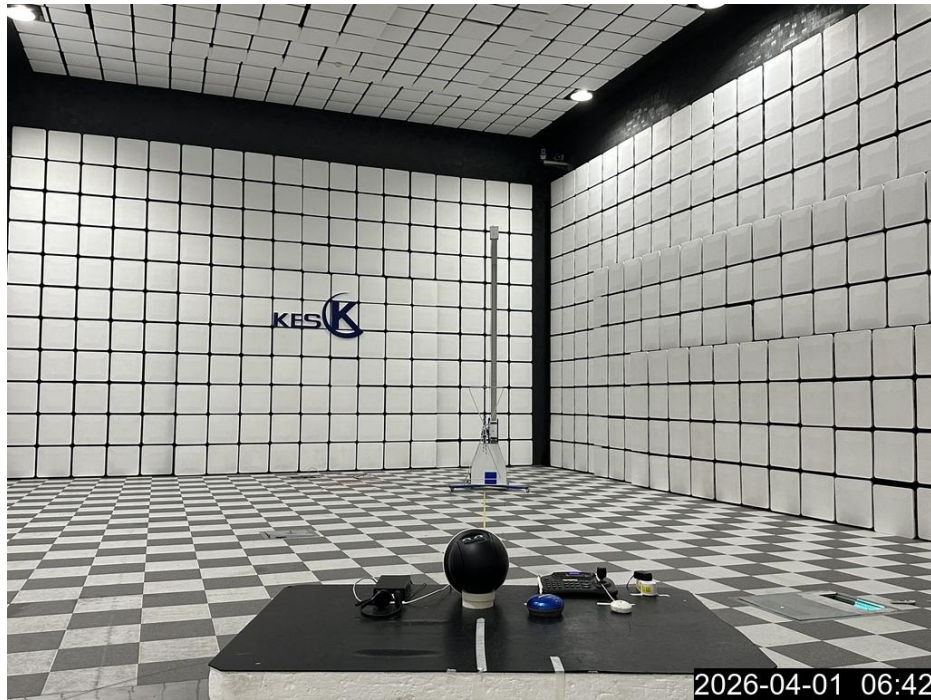
<방사성 방해-전면> Mode 2
