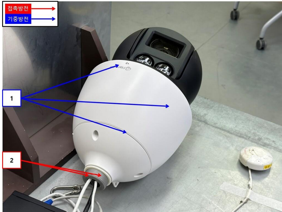
<정전기 인가부위-2> Mode 2
