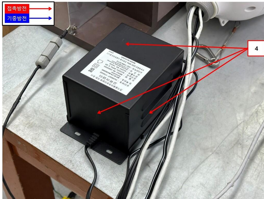
<정전기 인가부위-3> Mode 1
