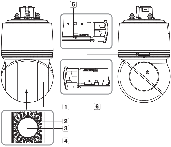
内部 (XNP-C9253R/XNP-C8253R/XNP-C6403R)
