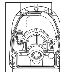
Крепежное отверстие
