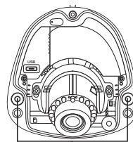
Крепежное отверстие
