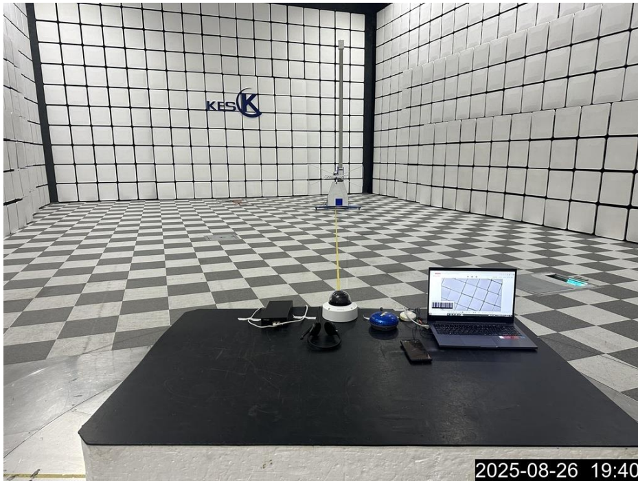
<방사성 방해-전면>
