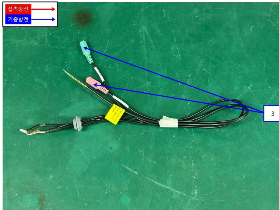
<정전기 인가부위-3>
