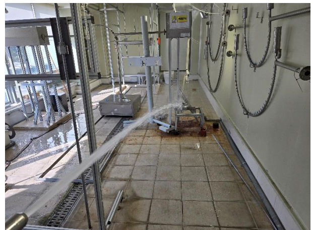
방수 시험
