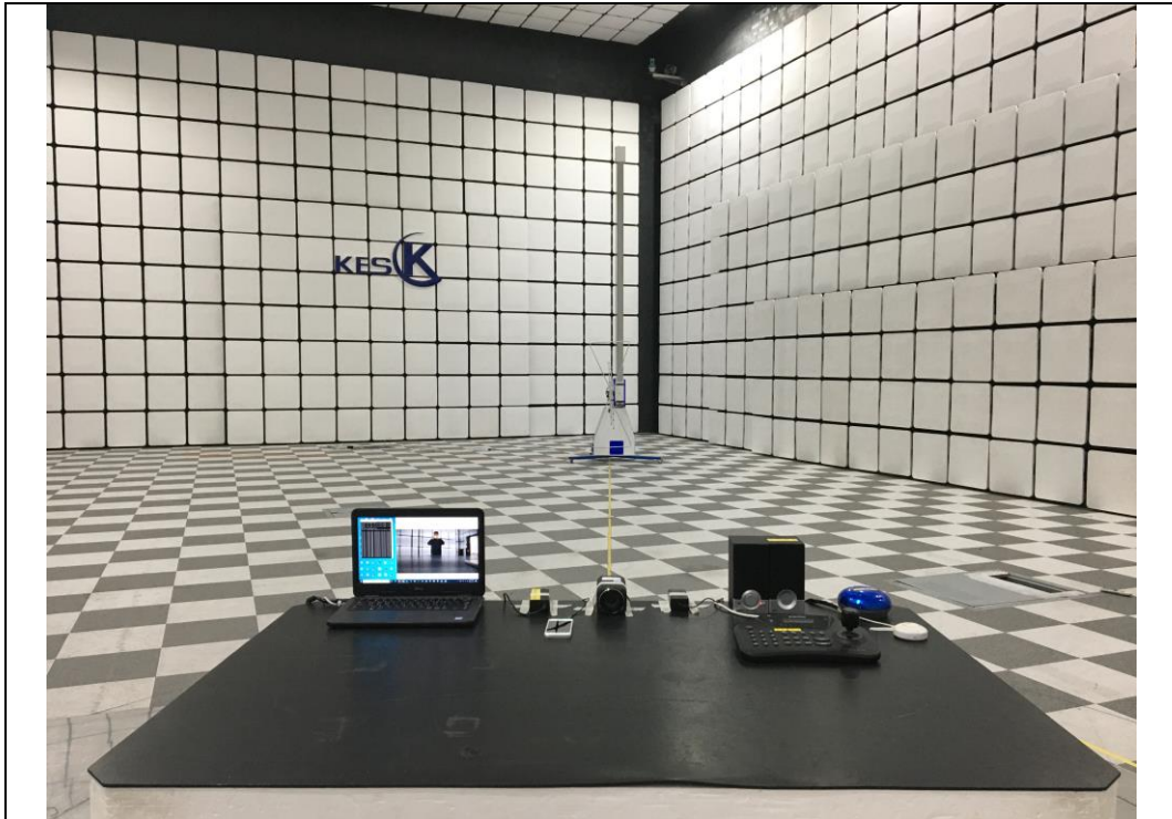
전 면 - DC Adapter 모드
