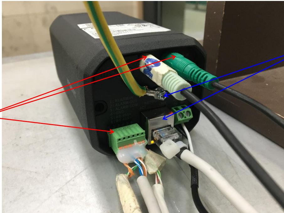
[시험기자재 - DC Adapter 모드]
