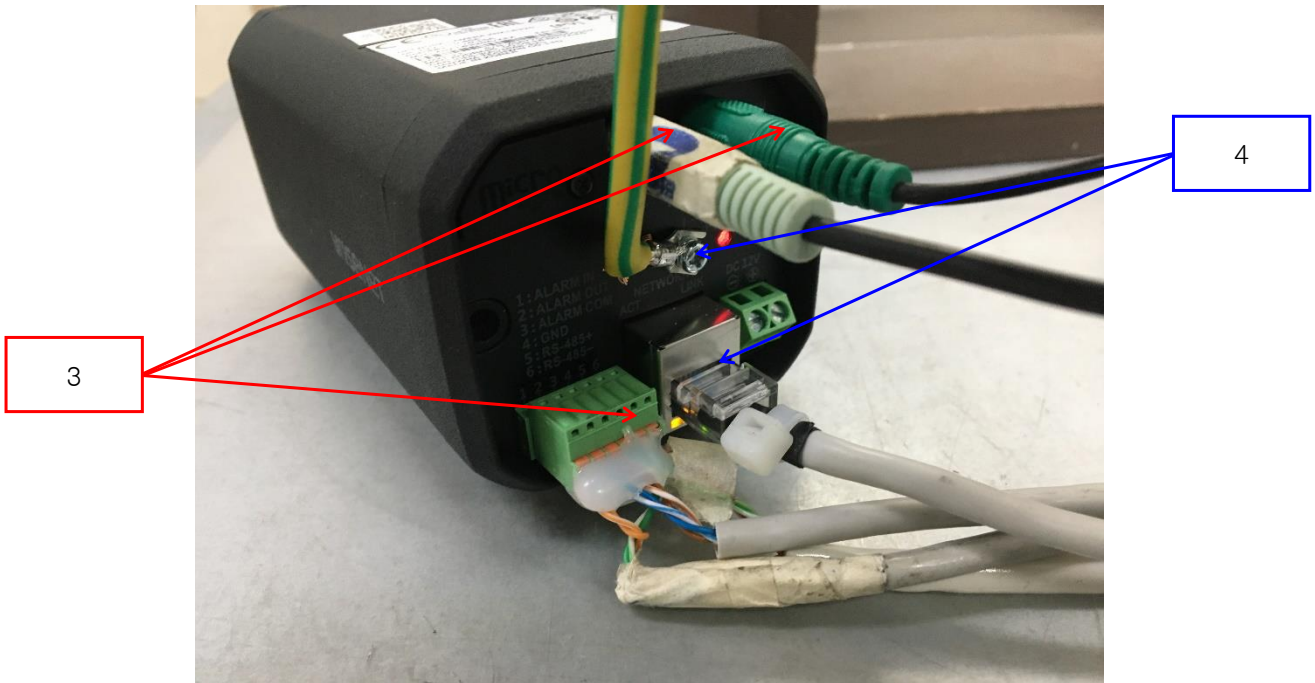
[시험기자재 - PoE Adapter 모드]
