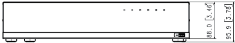
<XRN-2010/2010A>
