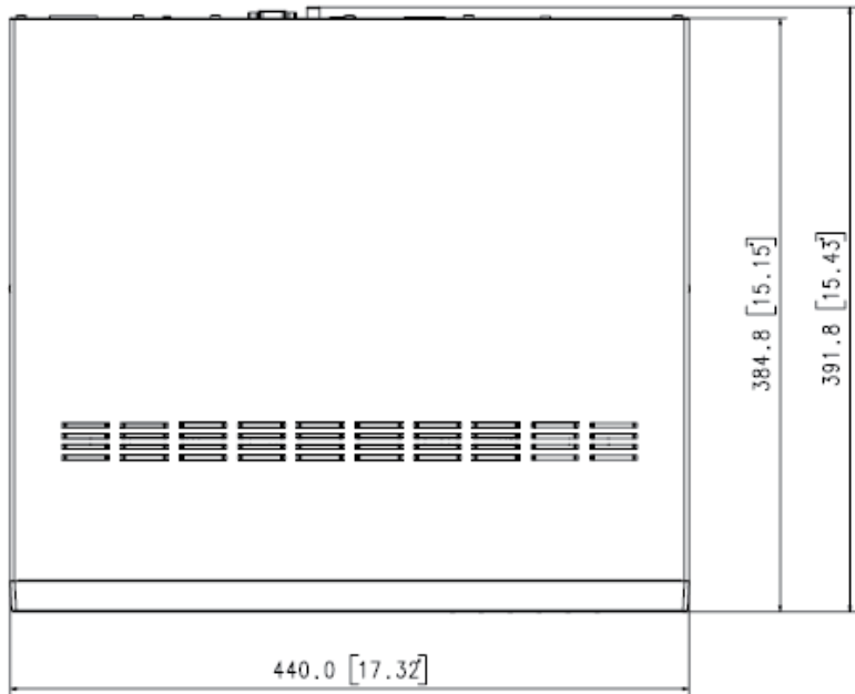
<XRN-2010/2010A>
