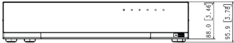
<XRN-2011/2011A>
