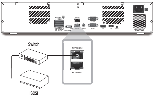
Er kan een switch gebruikt worden voor aansluiting
