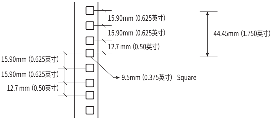
建议支架尺寸
