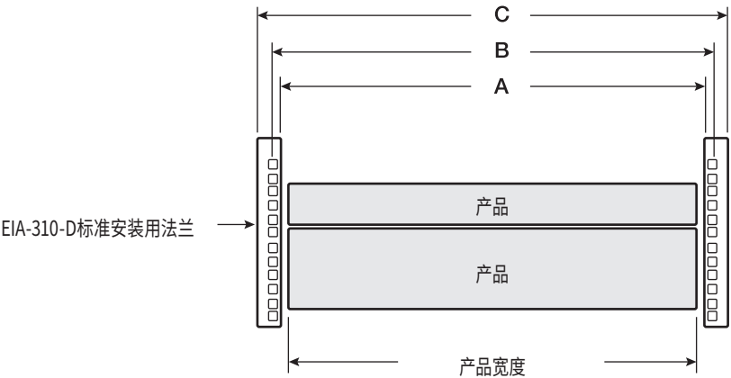
安装用法兰尺寸
